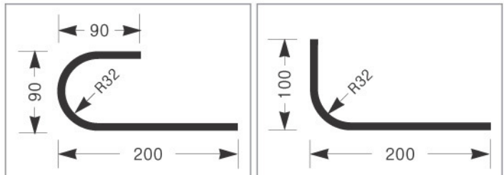
철근13mm 180° 절곡 (최소길이 320mm) 철근13mm 90° 절곡 (최소길이 270mm)
